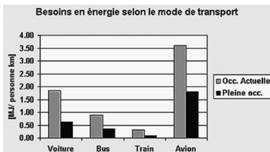
Besoin en énergie selon le mode de transport et le degré d'occupation des véhicules.
